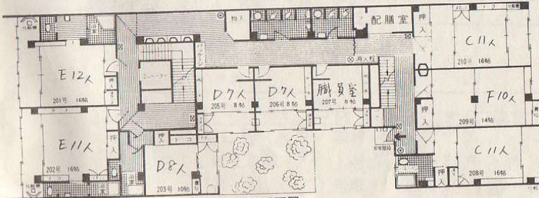
2階平面図
