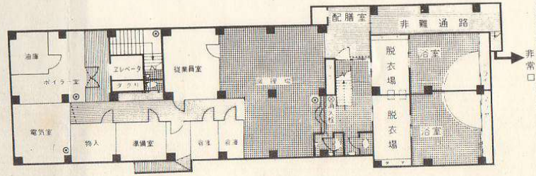
地階平面図
